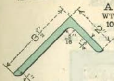
A. 149 WT. 6.2 LBS.
