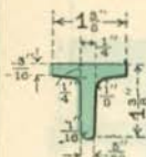
T. 189 WT. 1.9 LBS.
