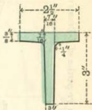
T. 185 WT. 1.5 LBS.
