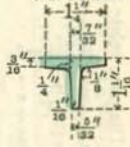
T. 185 WT. 1.5 LBS.
